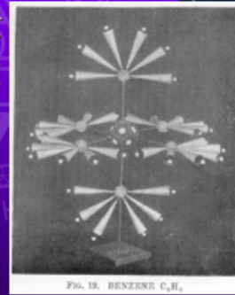
苯的模型 (benzene) C_6H_6
